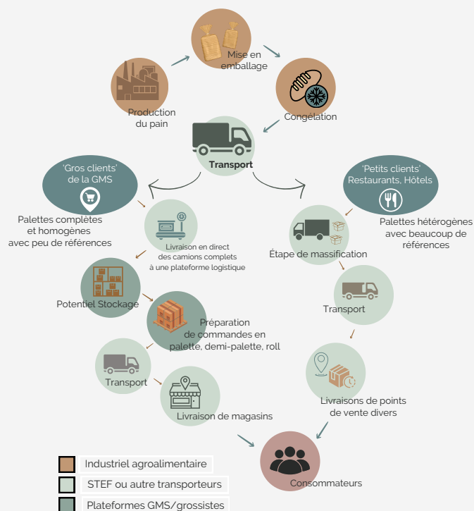
Figure 1 : Schématisation des activités industrielles liées au stockage et à la distribution de produits de boulangerie.
